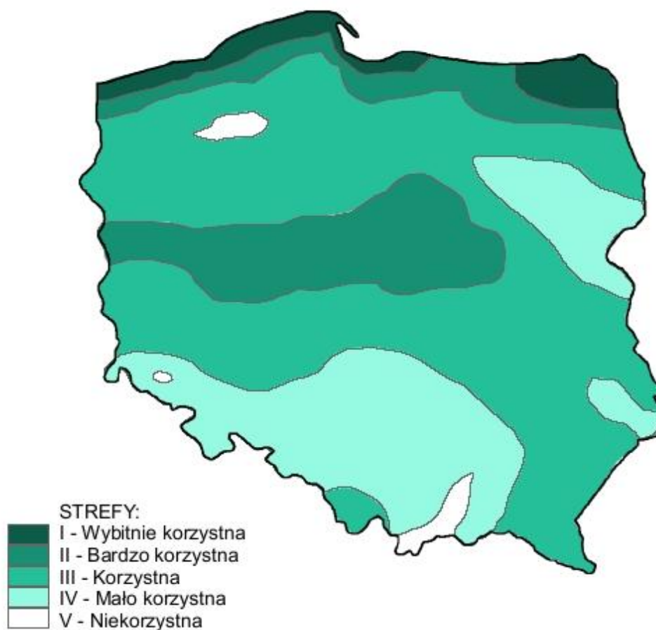
Rys. 18. Mapa stref energetycznych wiatru w Polsce
