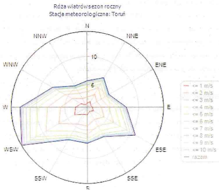
Rysunek 1. Róża wiatrów dla stacji meteorologicznej Toruń.
